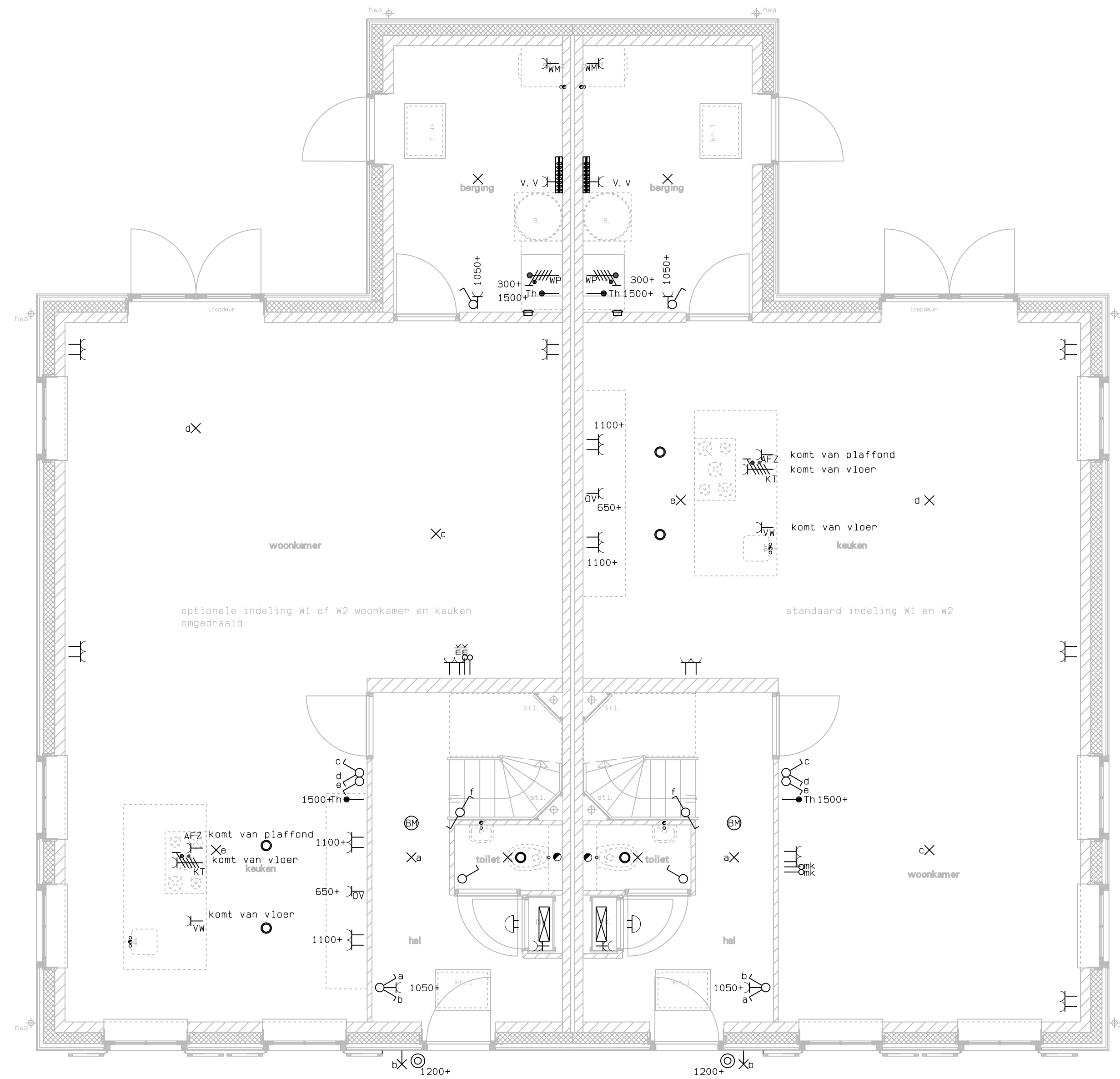
begane grond woning 1
