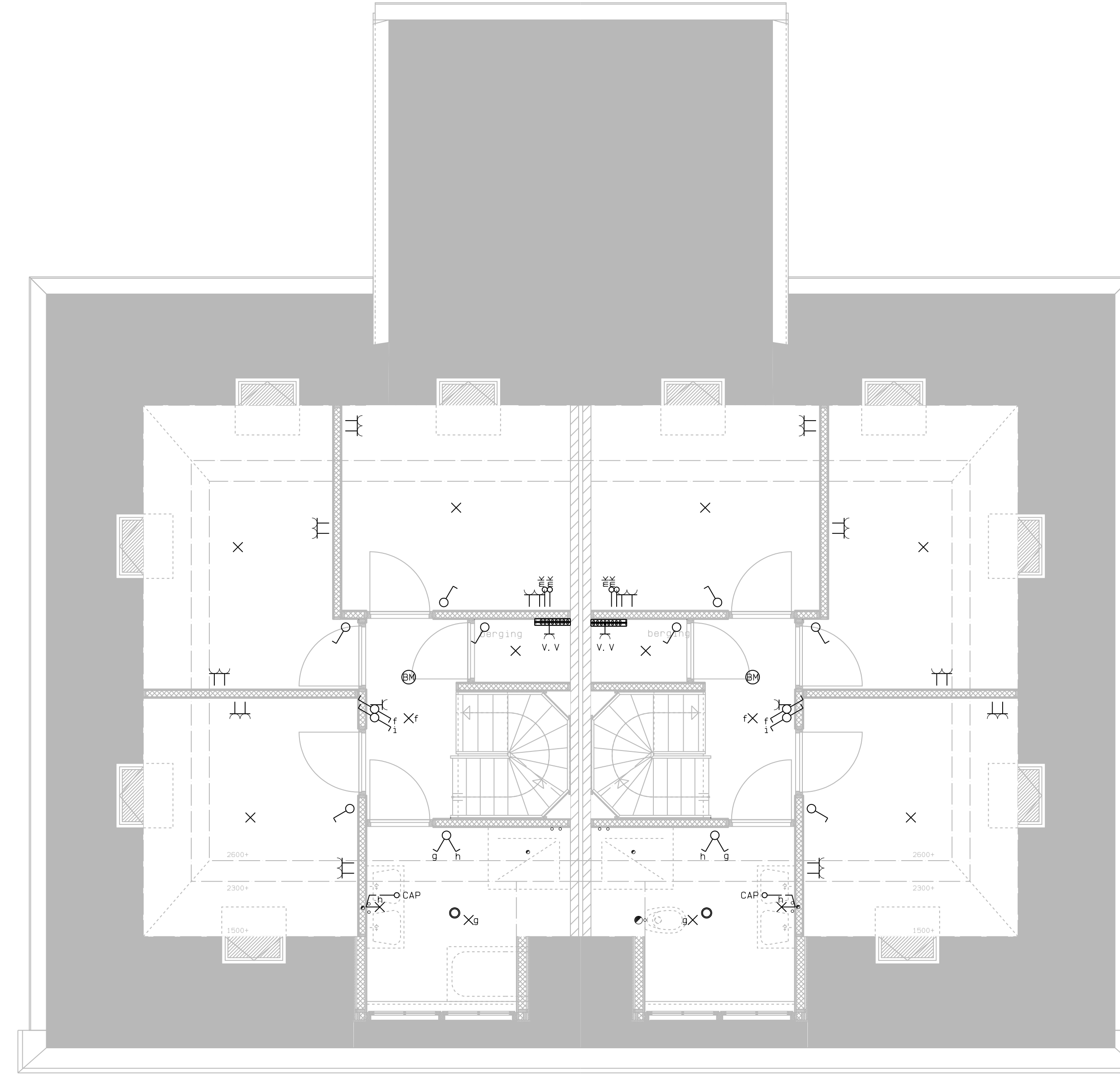
1e verdieping woning 1
